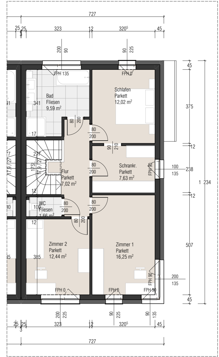
OBERGESCHOSS | 1:100
